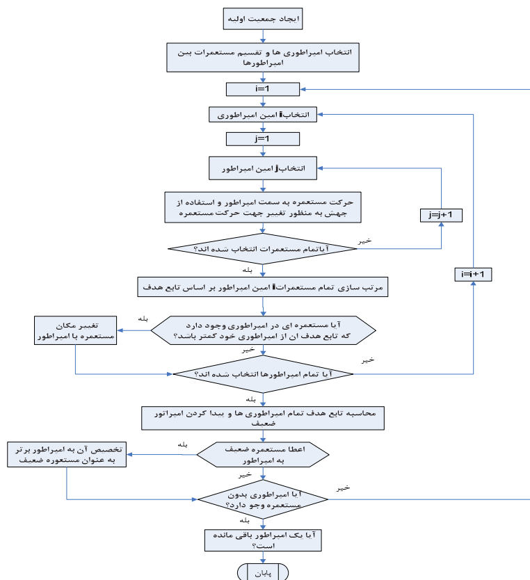
شکل ۲- نمودار جریانی مراحل الگوریتم ICA
